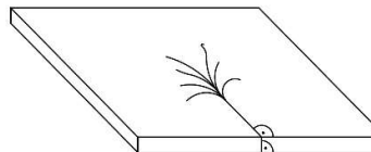
Thermischer Palm- od. Fächersprung
